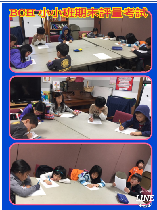
2019-Q4 Samal1Class
